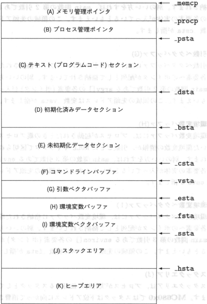
Fig. 7-1 ● プロセスメモリマップ
